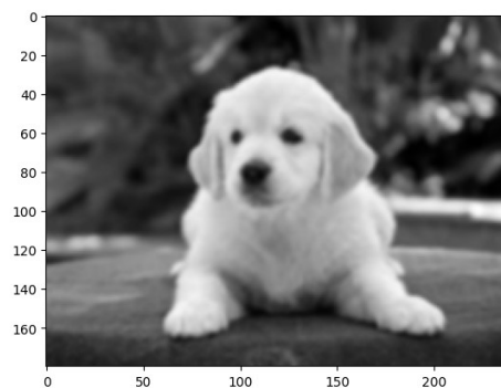
Blur
